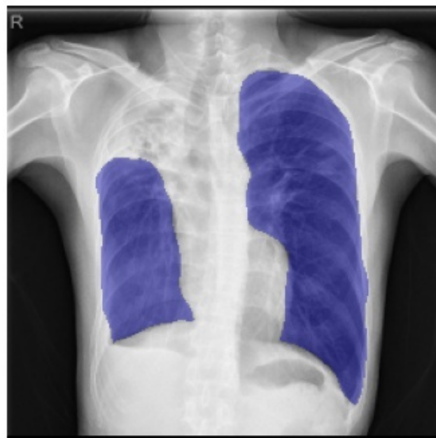
True Mask
