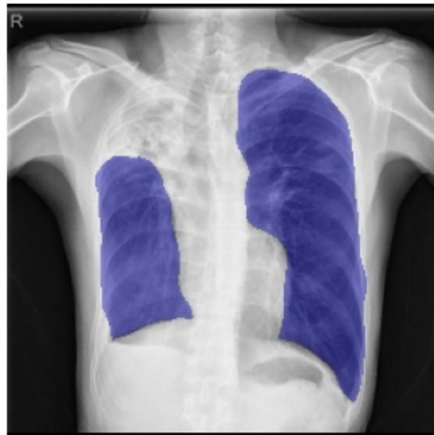
True Mask
