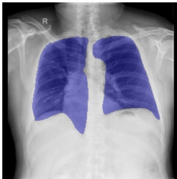
True Mask
