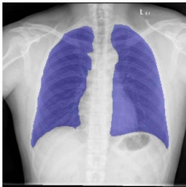
True Mask
